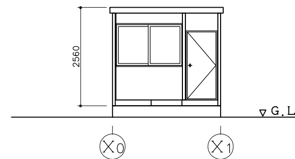
Y0通り立面図
