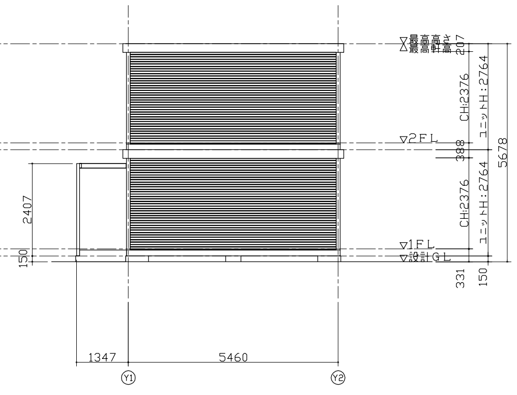
(X10) 通り立面図
