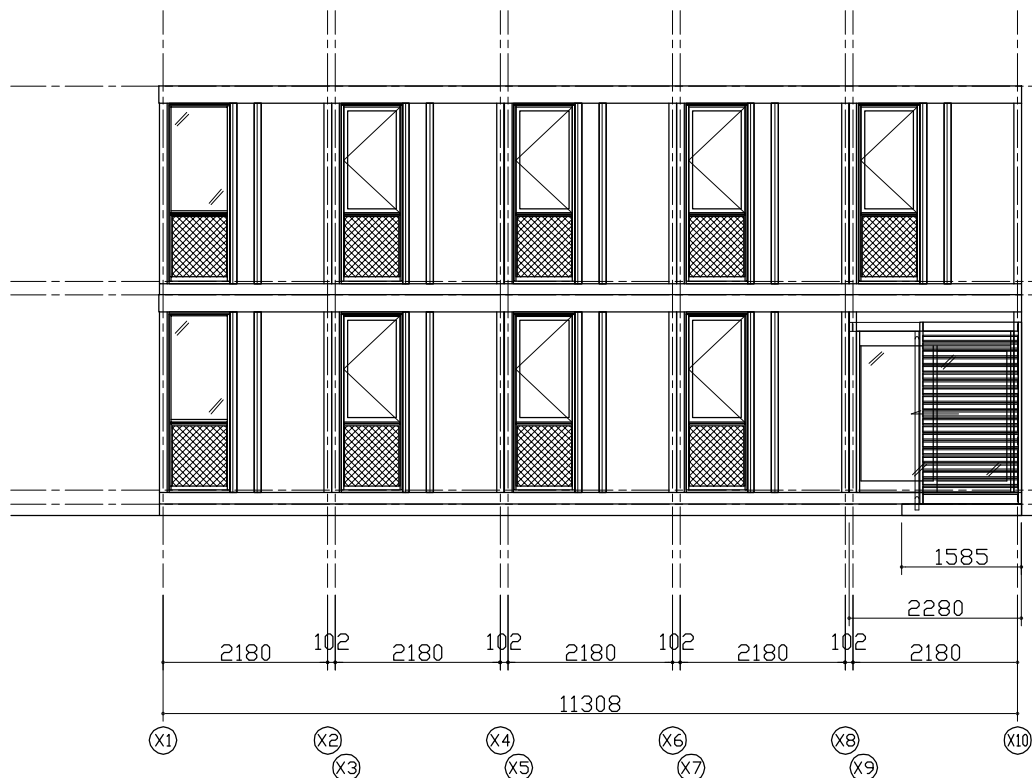
(Y1) 通り立面図
