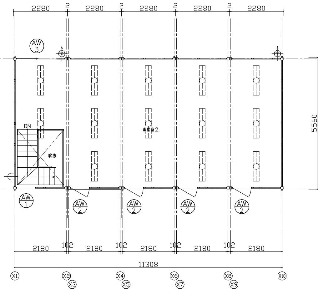
2階平面図
