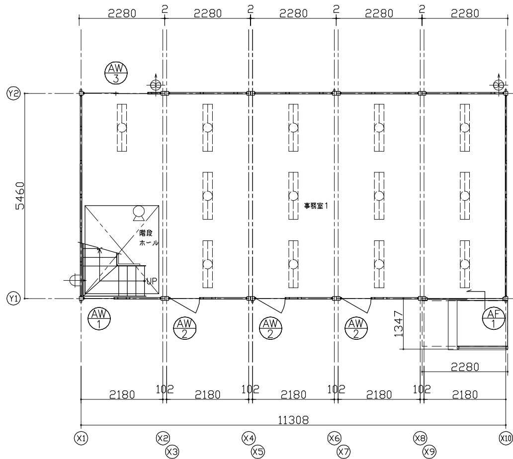
1階平面図
